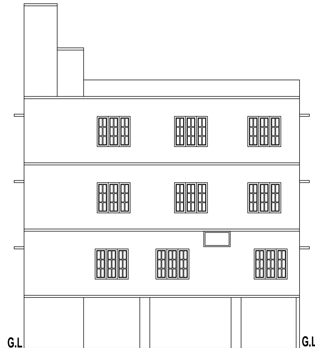
ELEVATION
